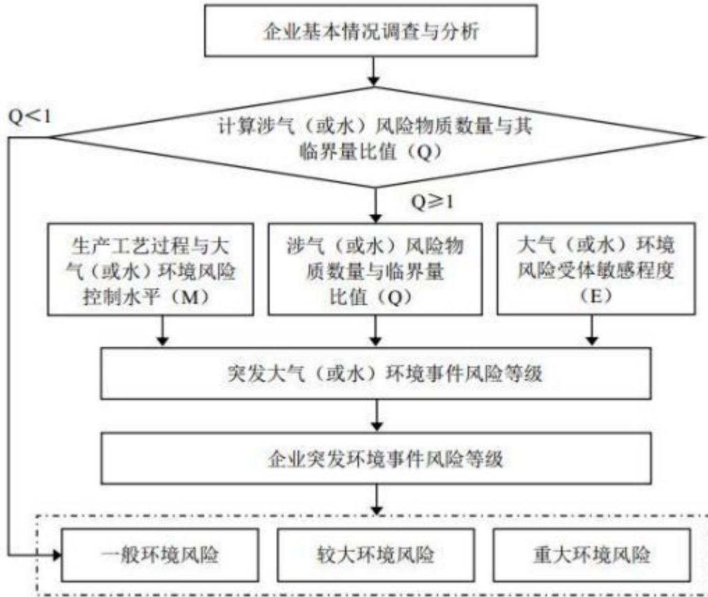
图 7-1 突发环境事件风险等级划分流程图
